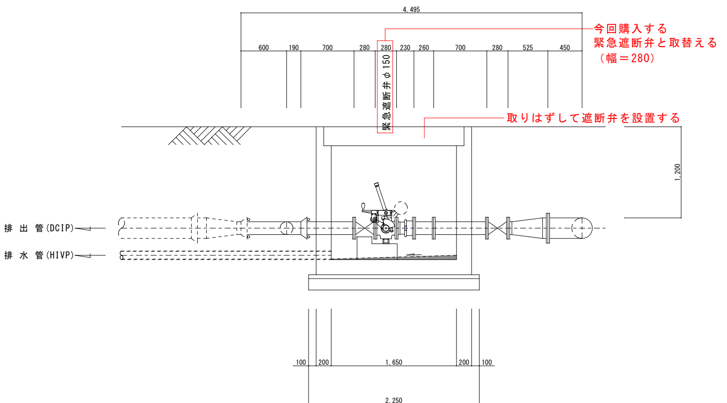
断面図
